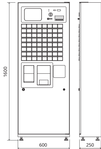
寸法図(単位:mm)
