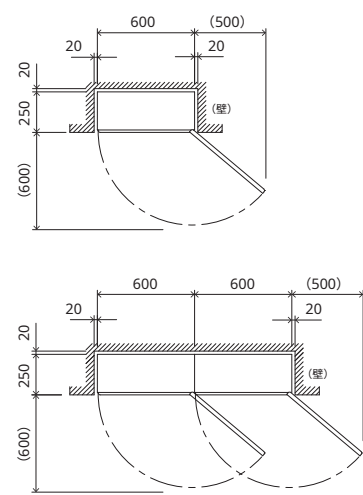
保守設置エリア図(単位:mm)
